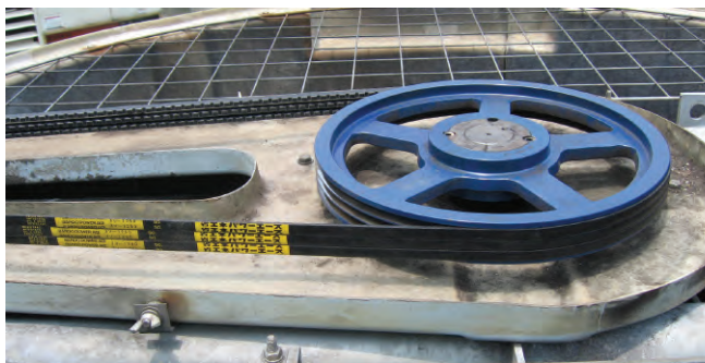
Vベルト (省エネパワーエース)
