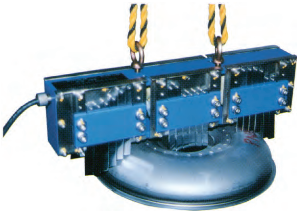
電磁マグネット
