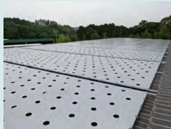
福岡県 | 倉庫 重ね式 1435.76 m 2
